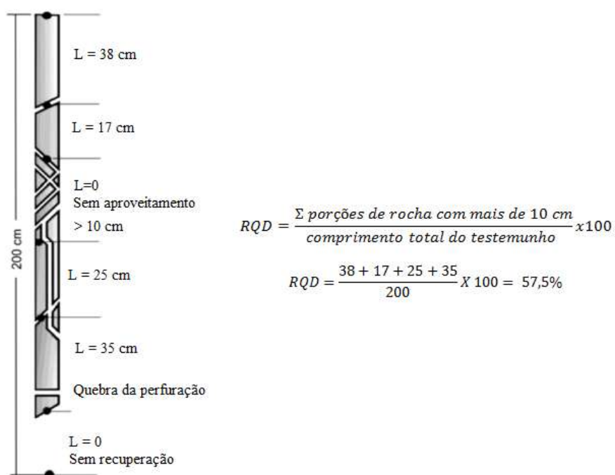
Figura 4 - Cálculo do RQD.
